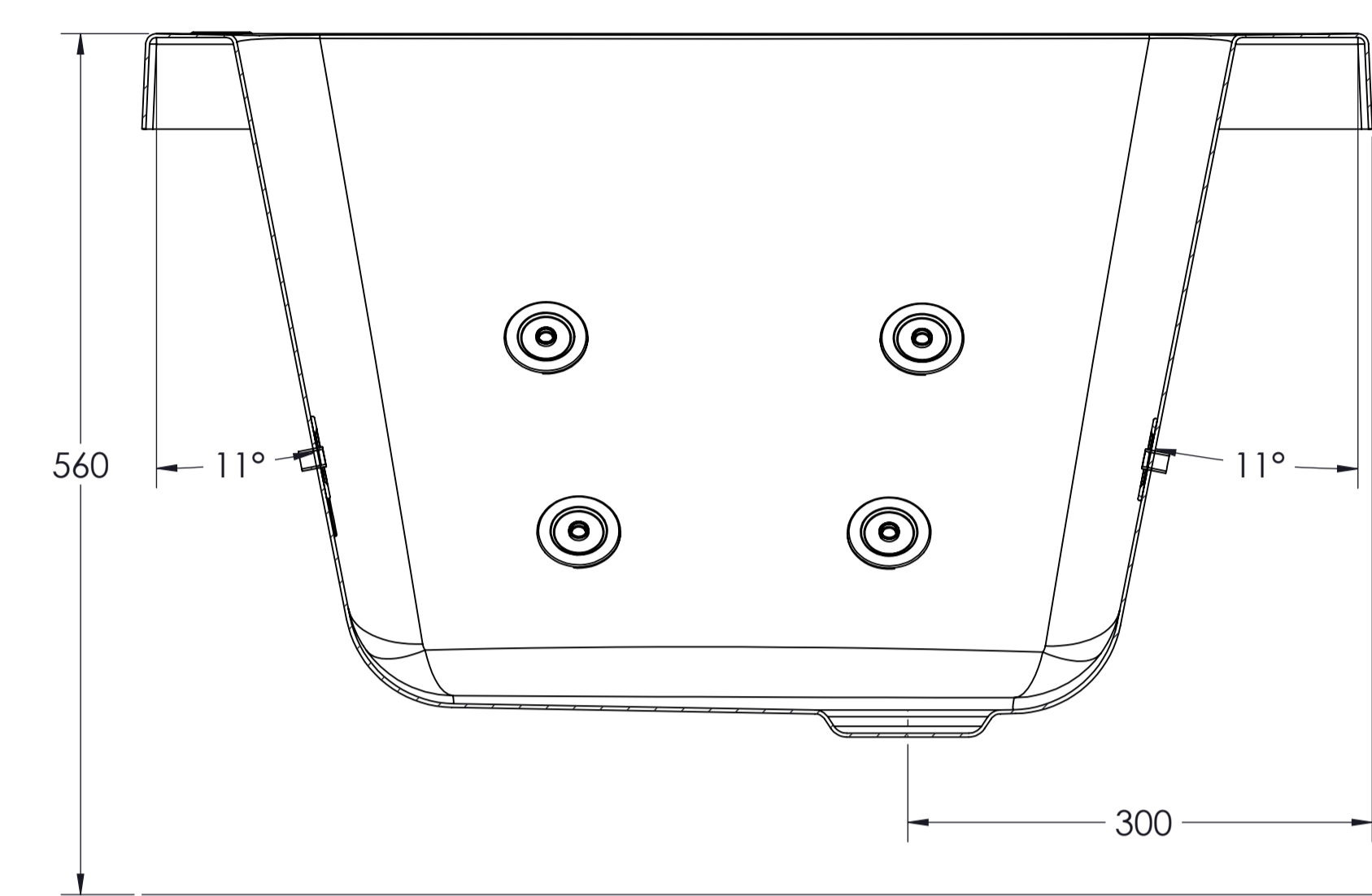
SECTION A-A
